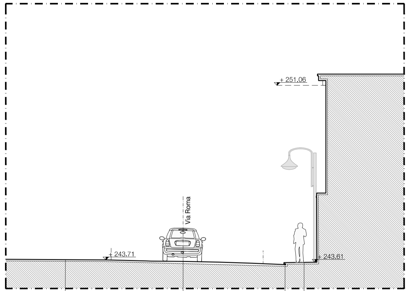
SEZIONE A scala 1/100
