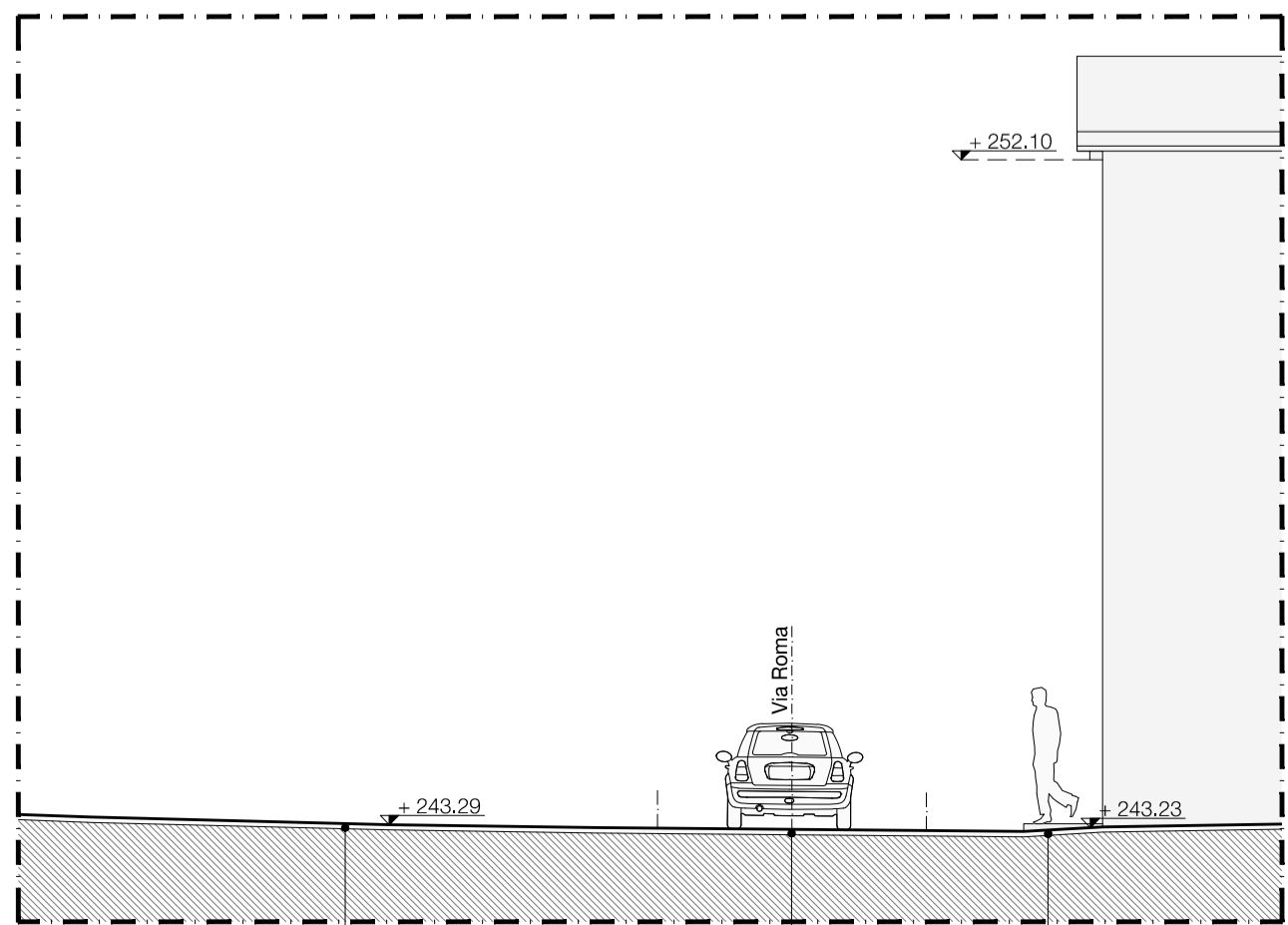
SEZIONE C scala 1/100
