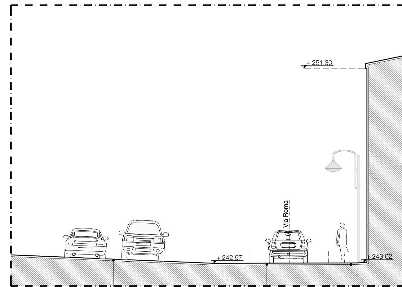
SEZIONE D scala 1/100
