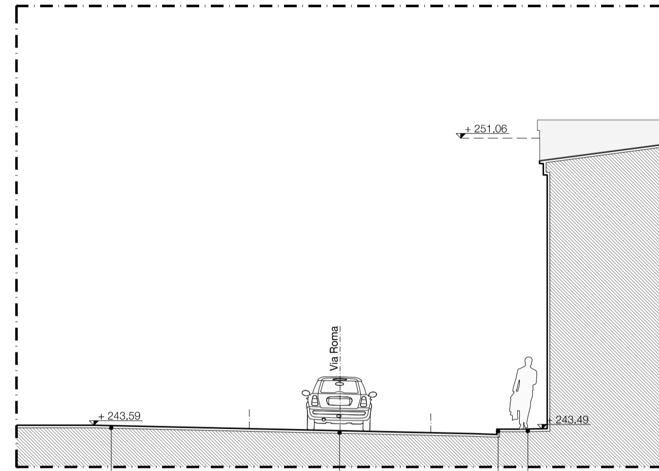
SEZIONE B scala 1/100
