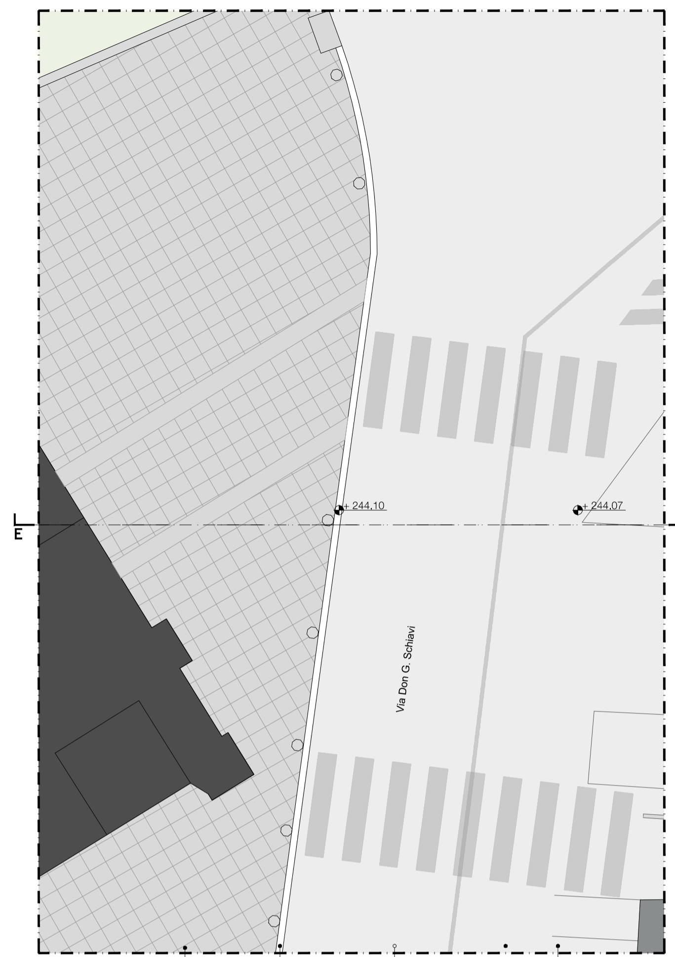
PIANTA E scala 1/100
