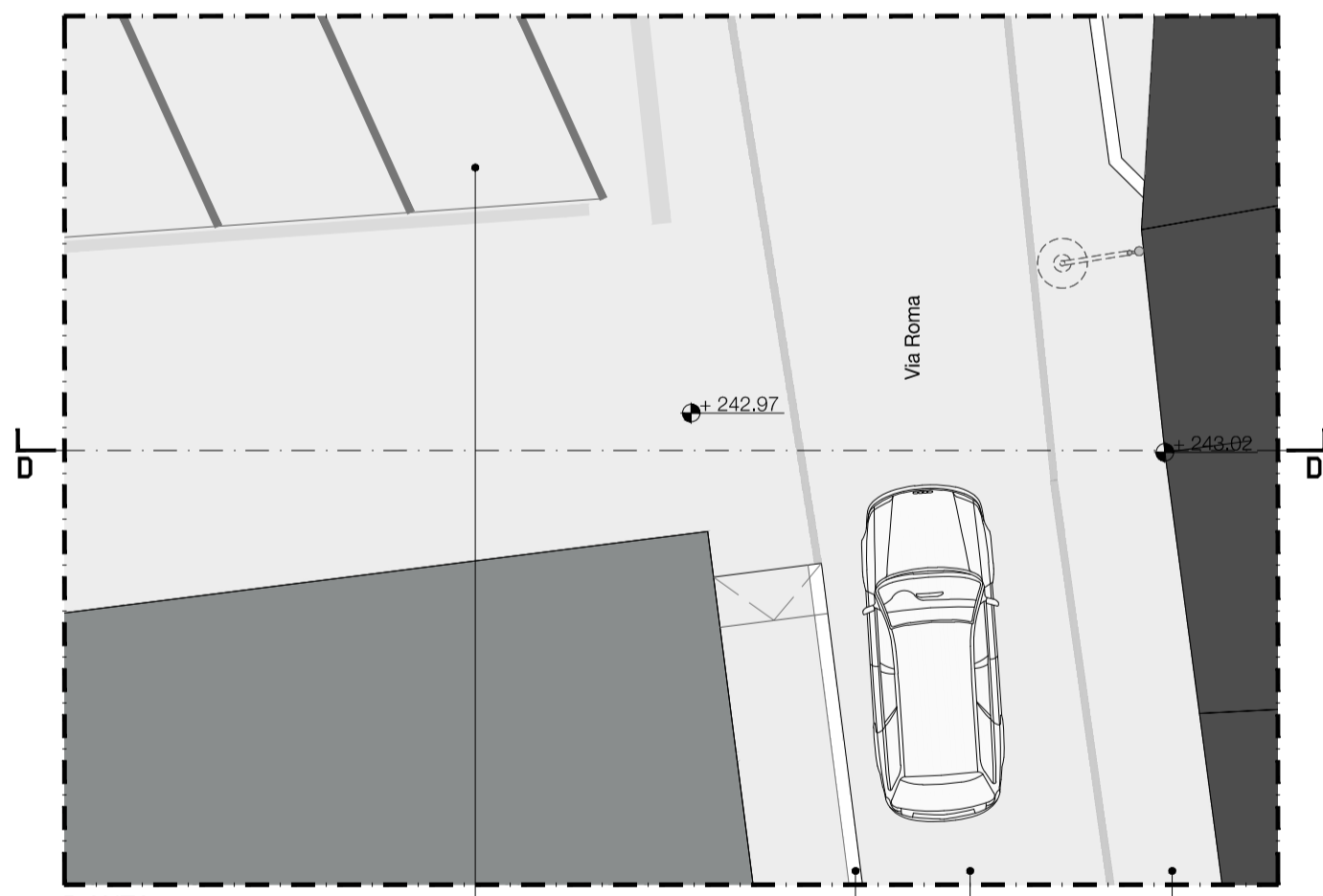
PIANTA D scala 1/100
