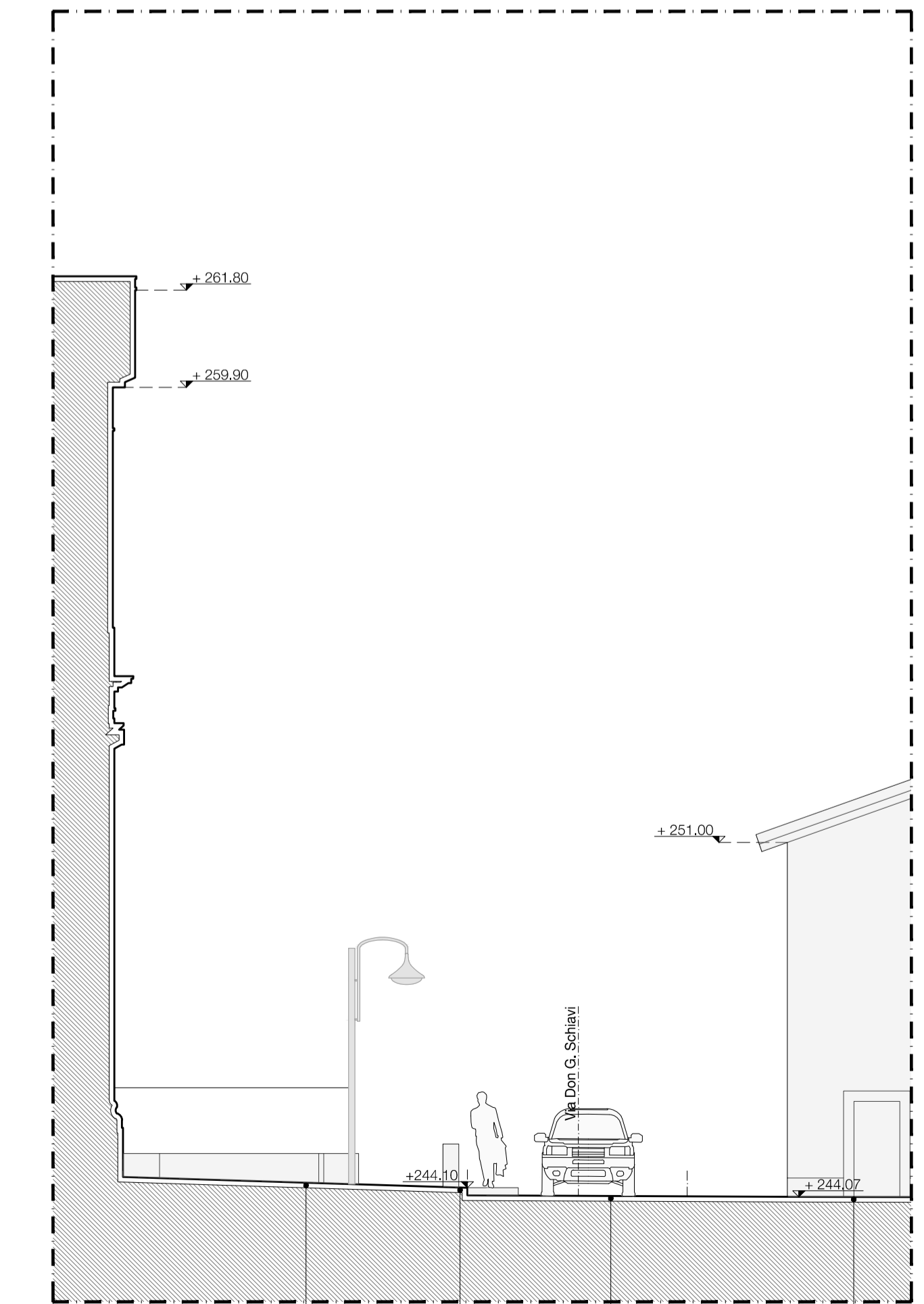
SEZIONE E scala 1/100
